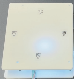
16 灯カラー LED による風向 / 風速表示ツール
