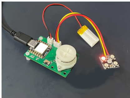
センサ専用基板 データ収集・無線通信機能 LED制御・LiPo電池対応
